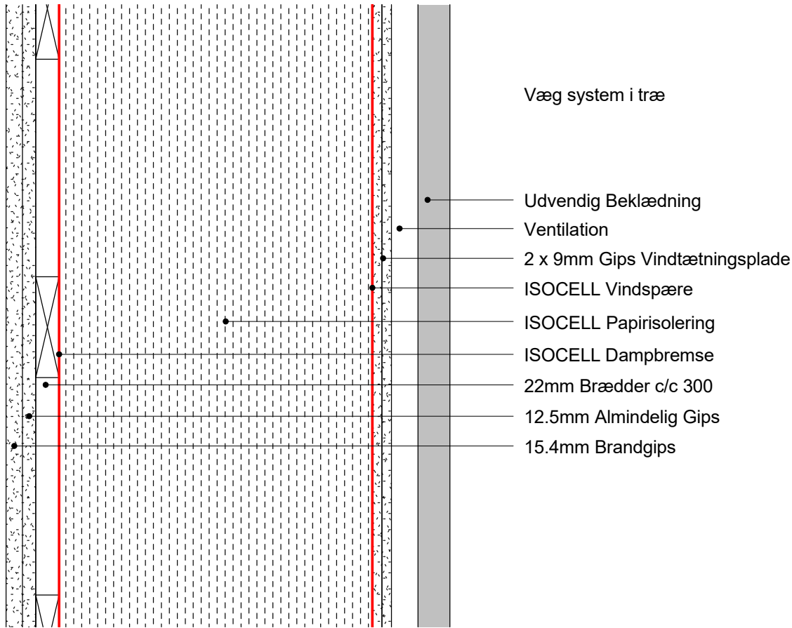
Målestok 1 : 5
